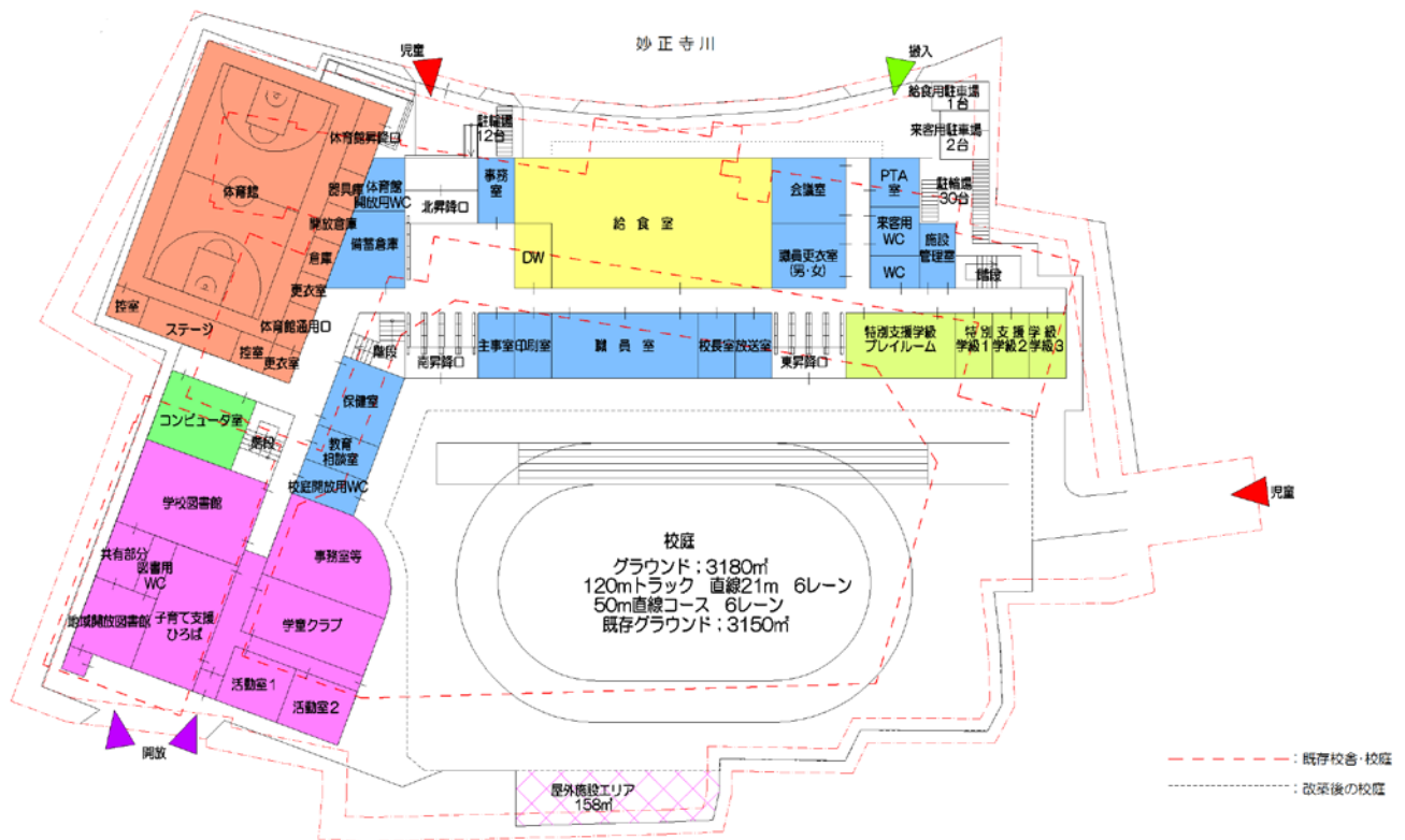
1階平面図兼配置図 (S=1/1000)
