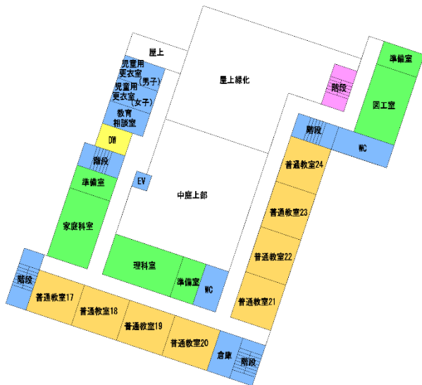
4階平面図 (S=1/1000)
