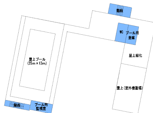
5階平面図 (S=1/1000)
