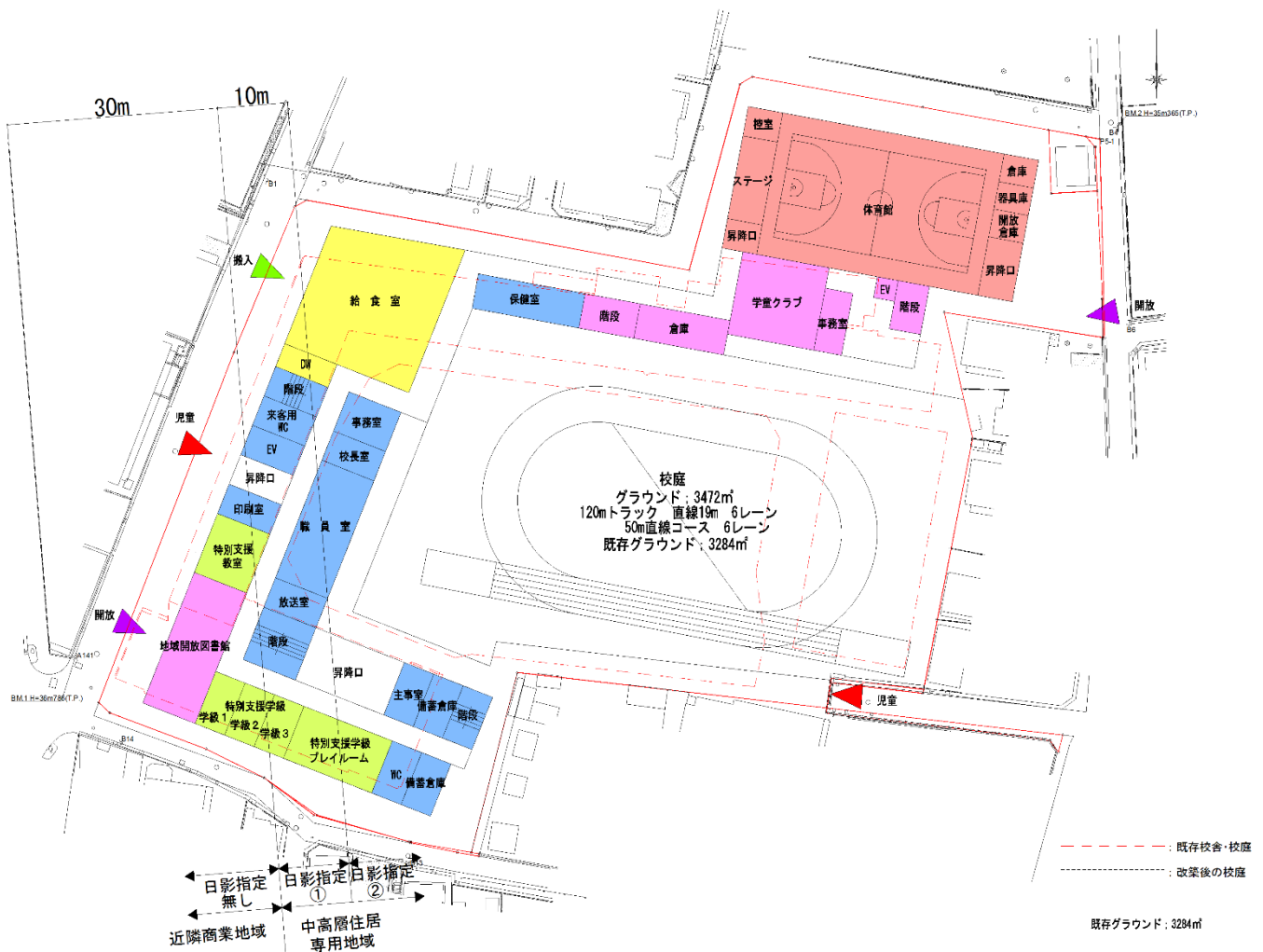
1階平面図 兼 配置図 (S=1/1000)
