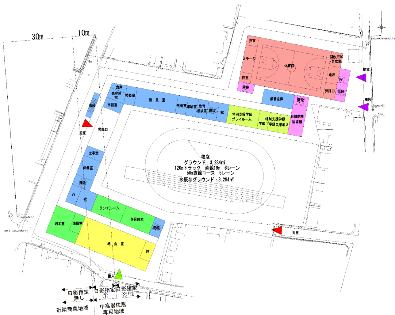
1階平面図 兼 配置図 (S=1/1000)
