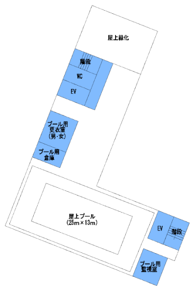
5階平面図(S=1/1000)
