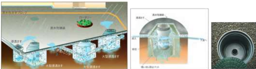
図 6-5. 公共施設前広場の浸透施設設置イメージ断面図（左） と浸透ますの構造図（中央）と写真（右）
