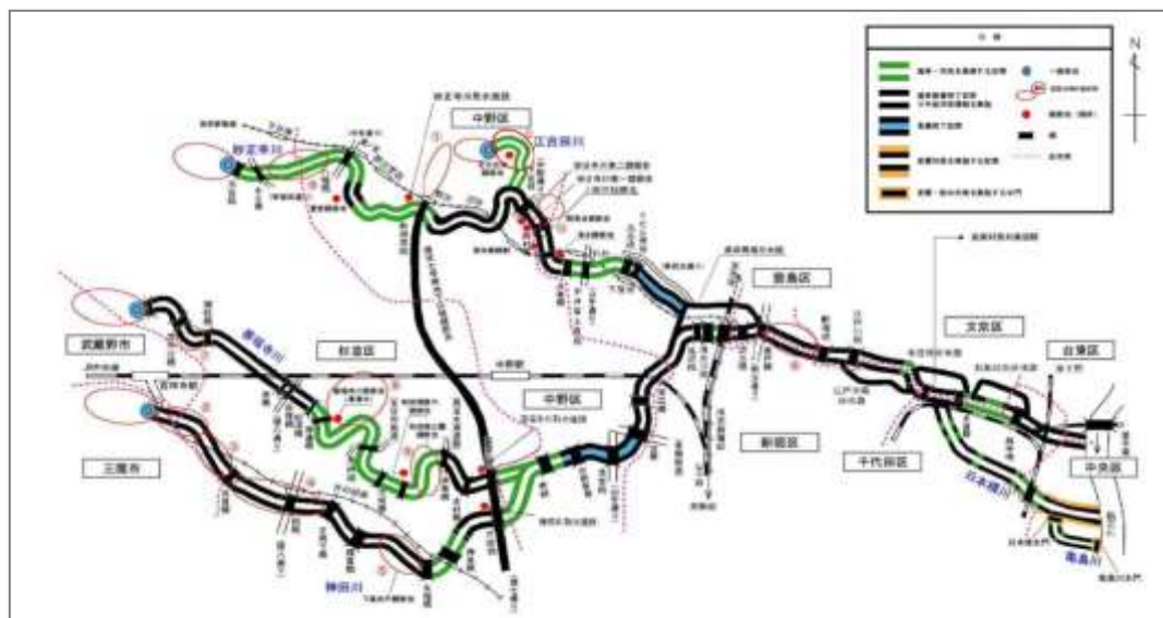
図 3-4. 神田川流域河川整備箇所図と凡例拡大図
