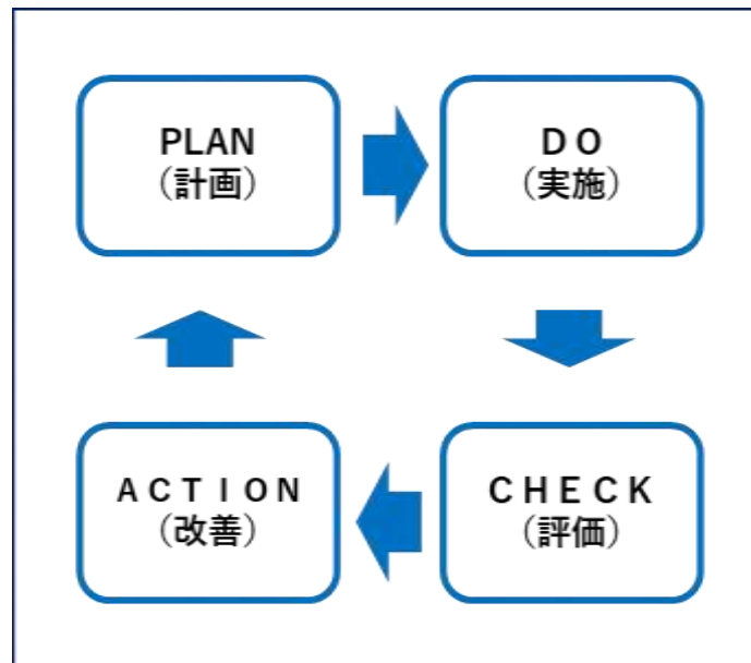
図 7-1. PDCA の図
