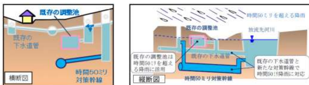
図 3-5. 50mm 拡充対策の下水道設備の具体的取組—既存設備を活用した施設整備の例
