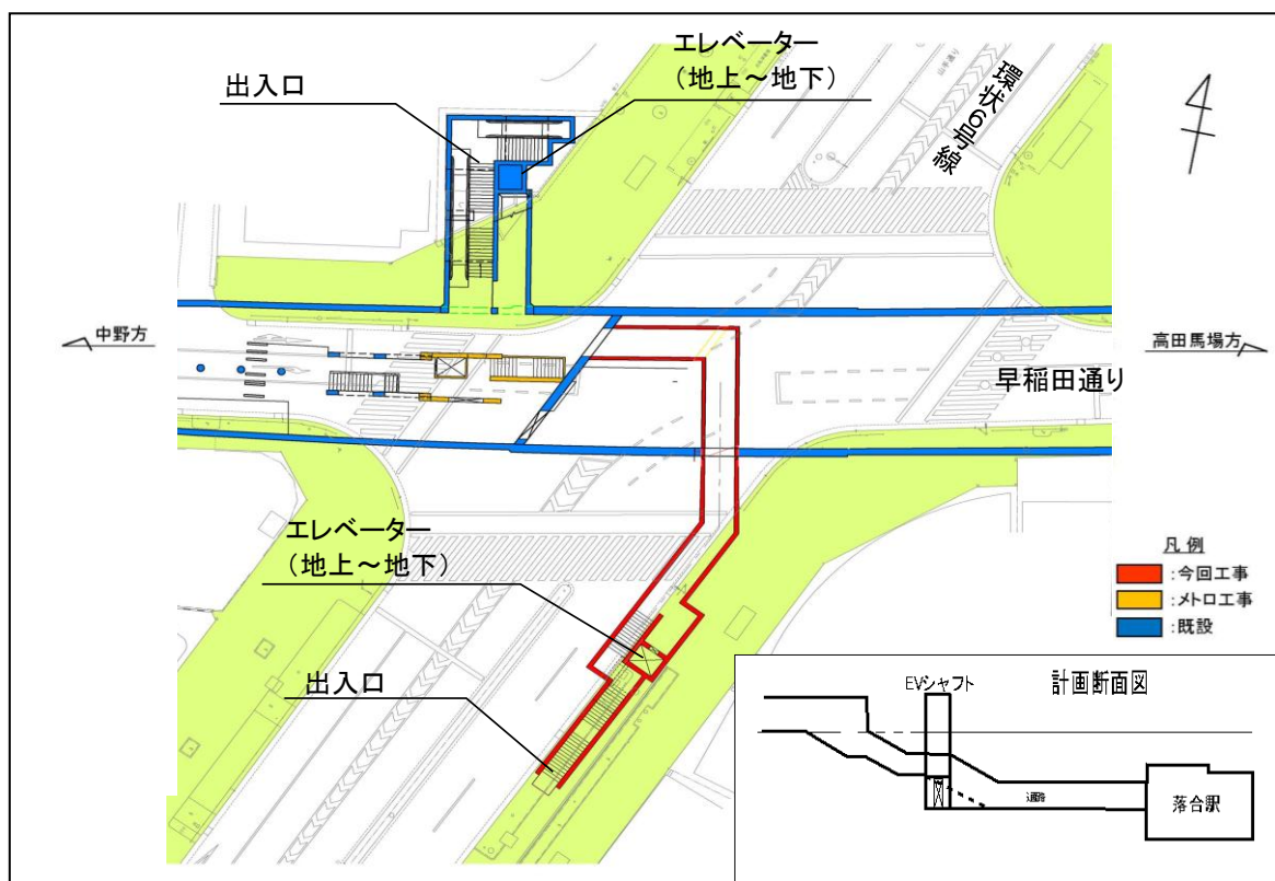
【地下横断通路計画図】
