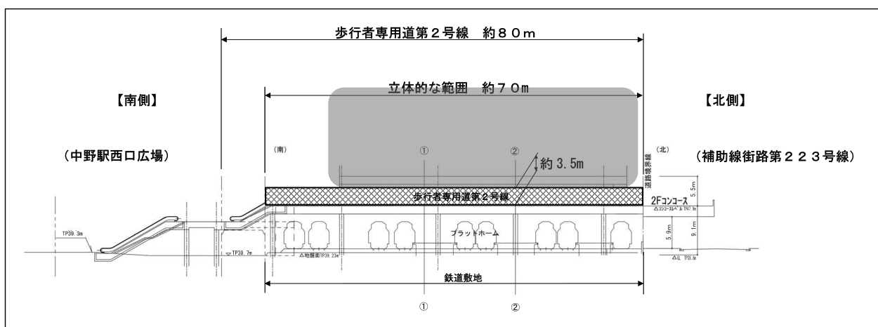
【縦断面図】
