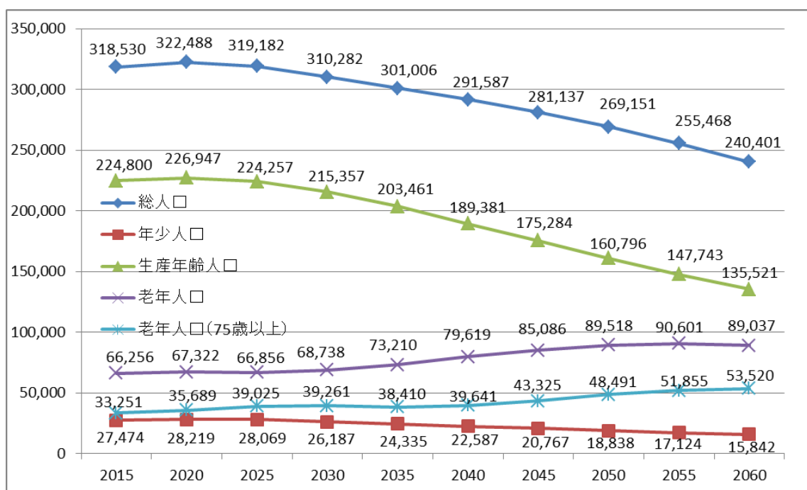
【図 7】基本推計
