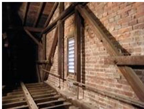
写真10 天井裏小屋組（裏面西側）
