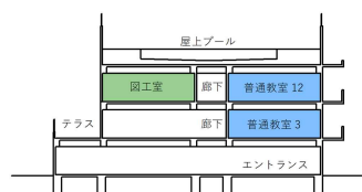
B-B' 断面図(S=1/800)
