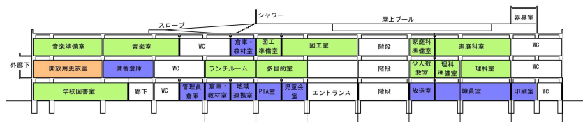
C-C' 断面図(S=1/800)
