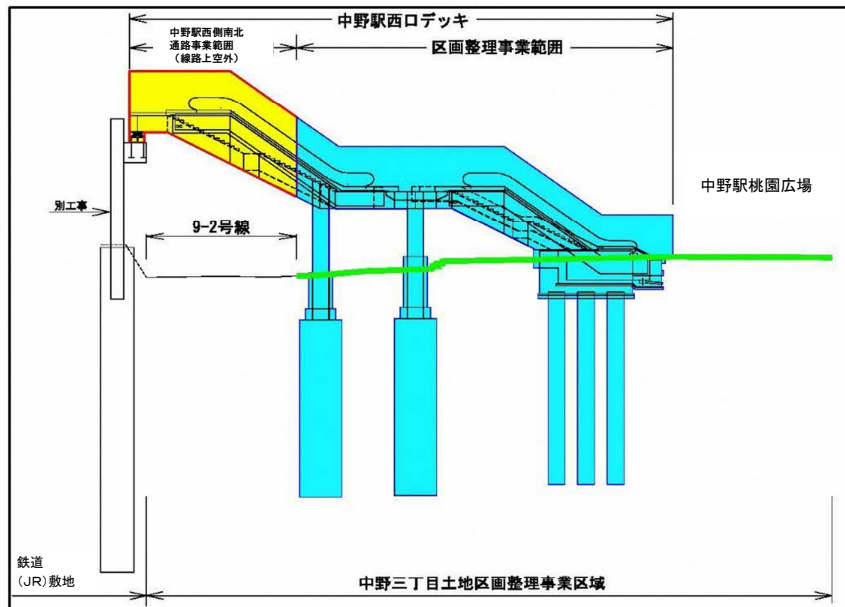
A-A断面図
