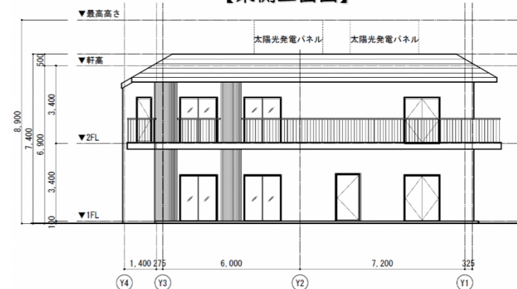
【西側立面図】
