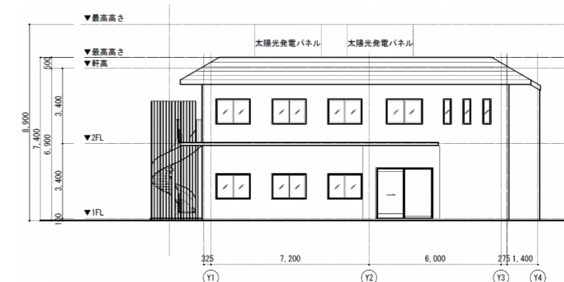
【東側立面図】
