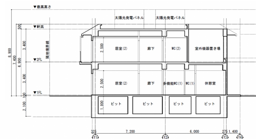
【B-B 断面図】
