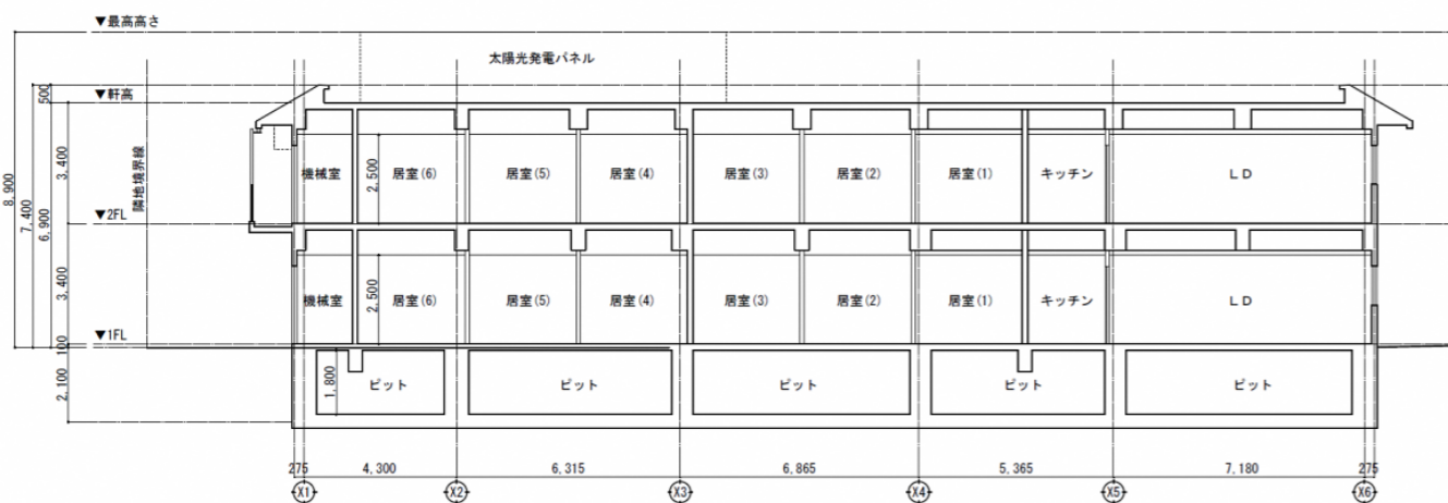
【A-A 断面図】
