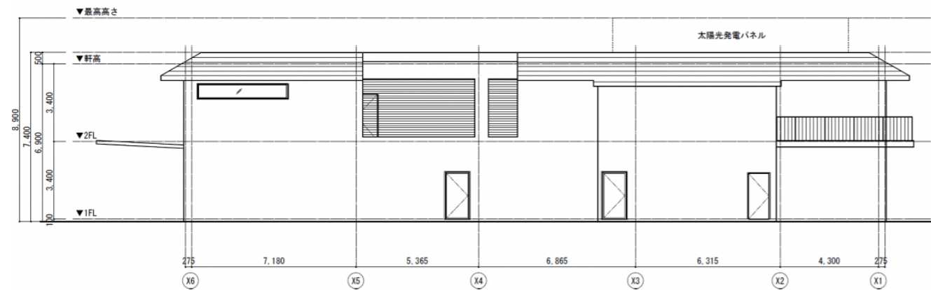
【北側立面図】
