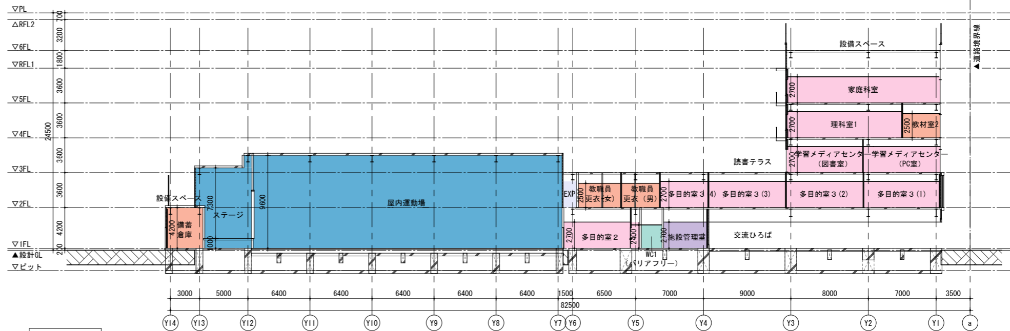
B-B' 断面図
