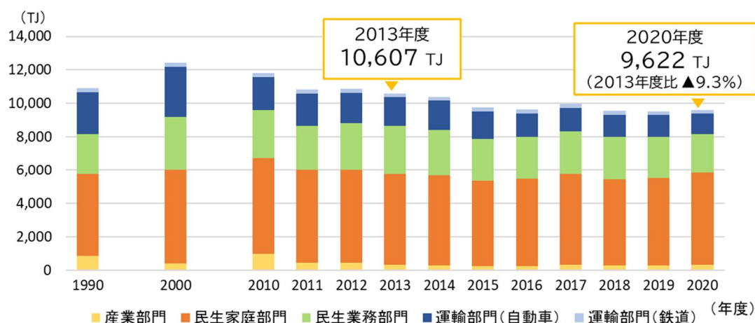
エネルギー消費量の推移
