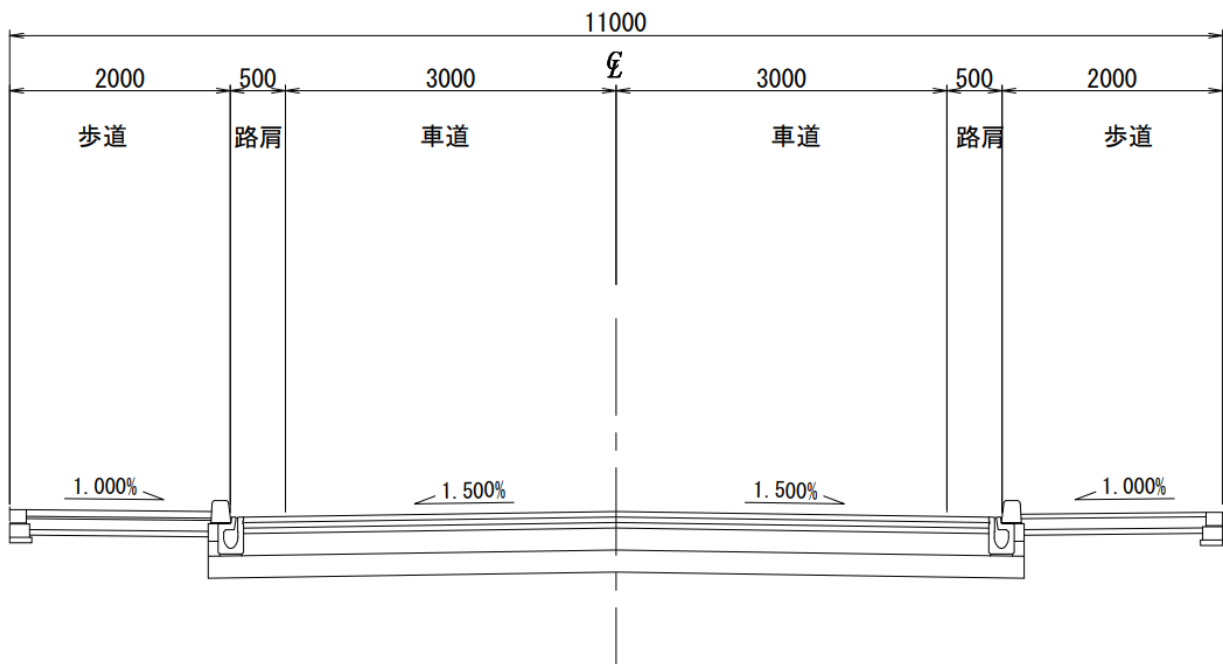
横断面図
