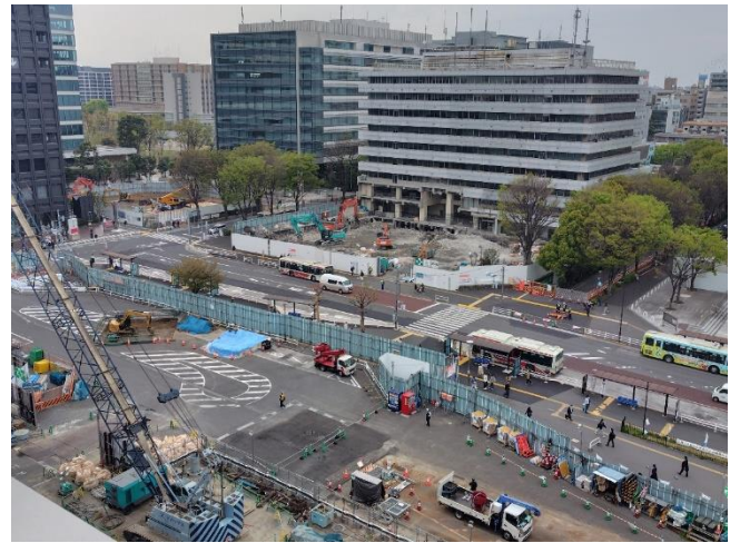
ペデストリアンデッキ下部工の基礎工事の状況
