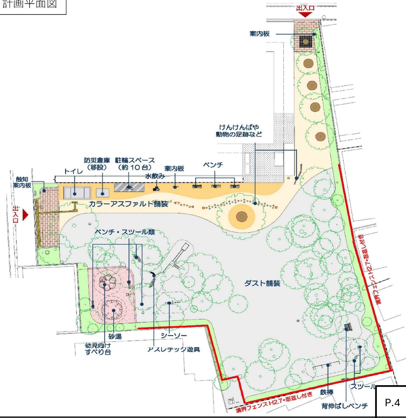
計画平面図
