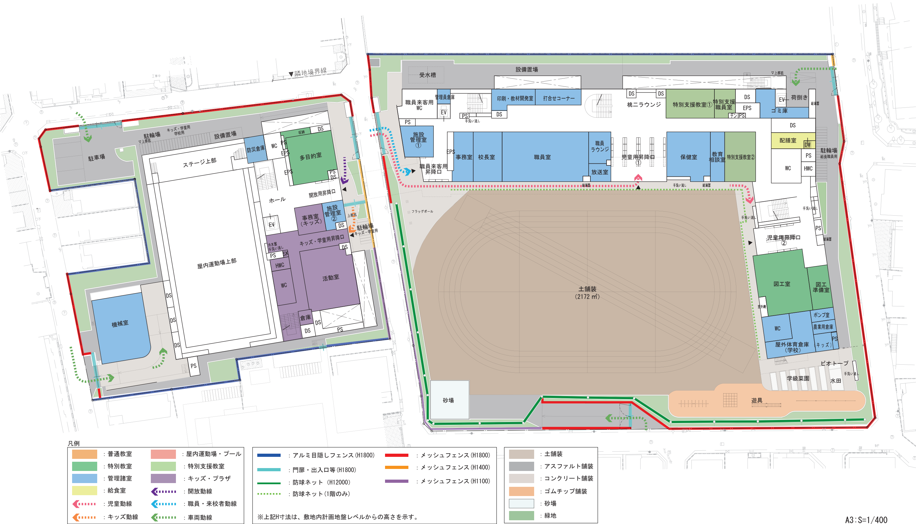
平面図（配置図・1階）
