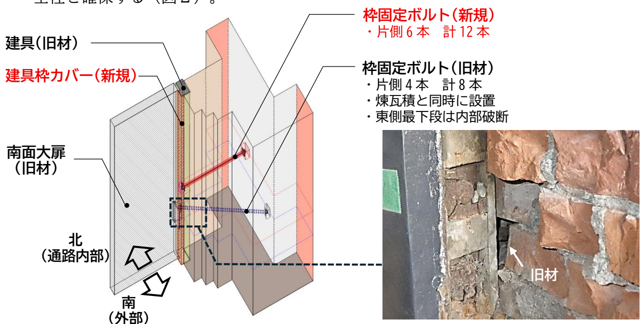
図2 南面木製大扉修復イメージ図
