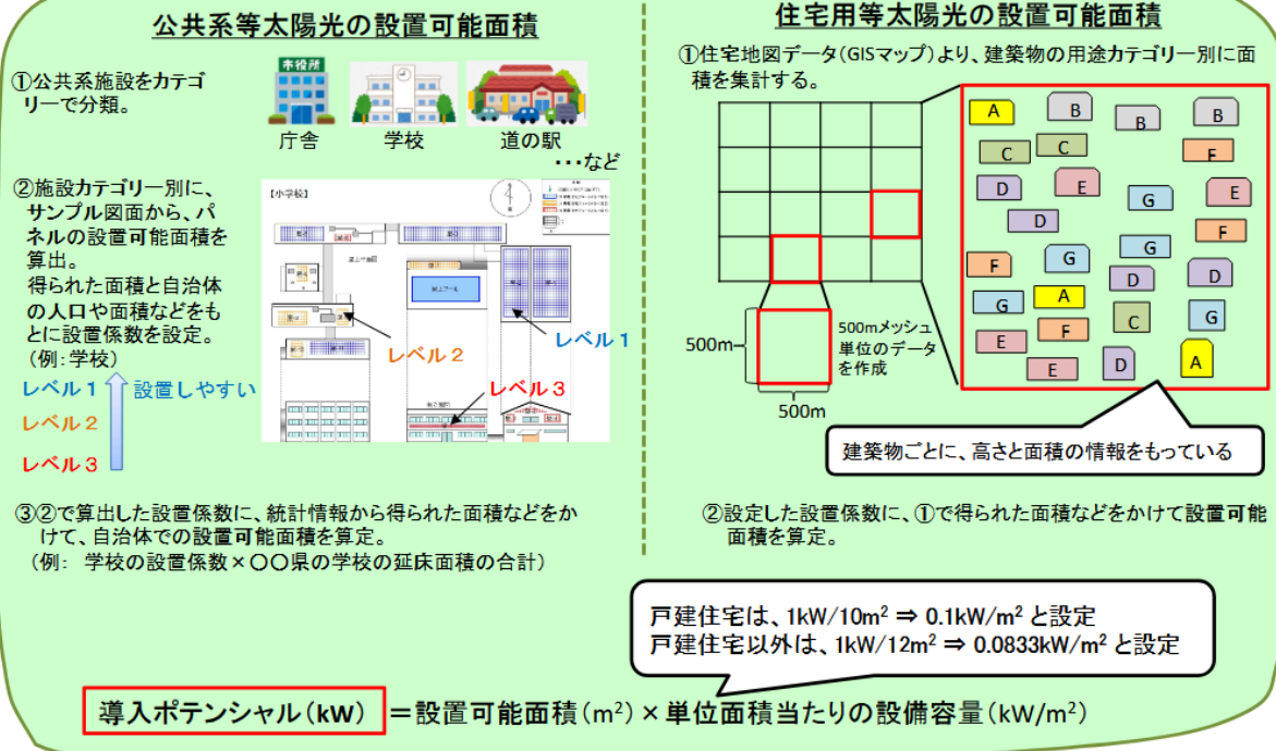
図6 REPOS における太陽光導入ポテンシャルの算定方法
